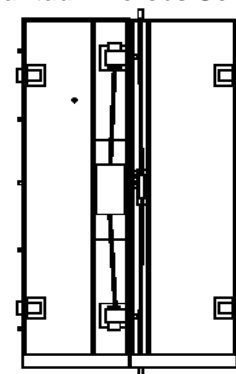
Vantaux Tiercés Sol. 4
